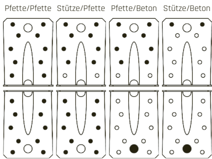
TYP 65/90S 1,5 GREENLINE mit Steg 6503S15
