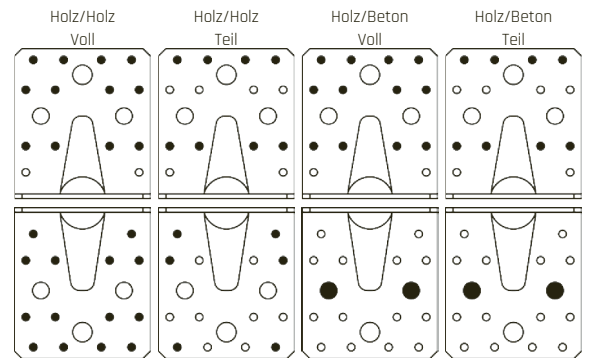
KR Rundloch 135 mm 1101353 / 110135
